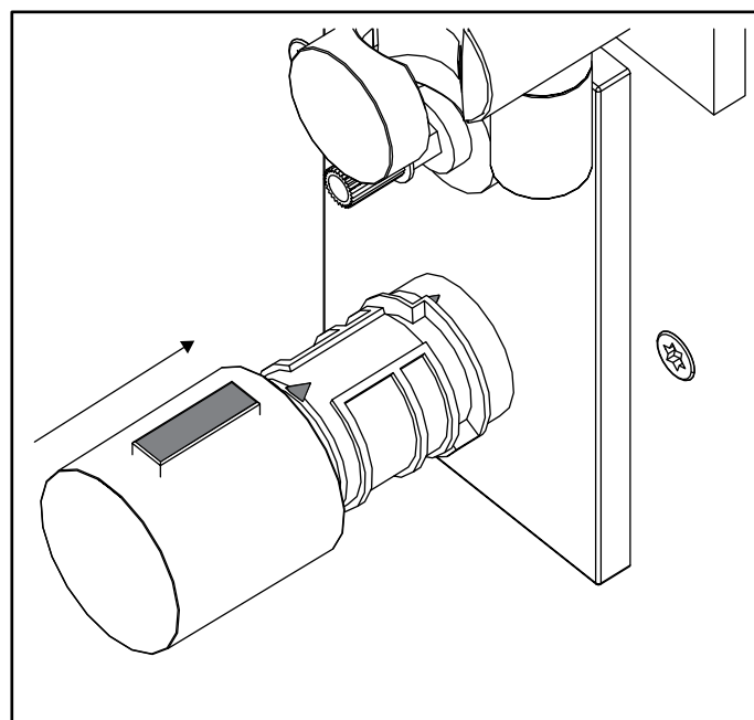
Fig. 14 Tryck på termostadvredet. Obs! Tänk på att pilarna ska vara uppåt.
