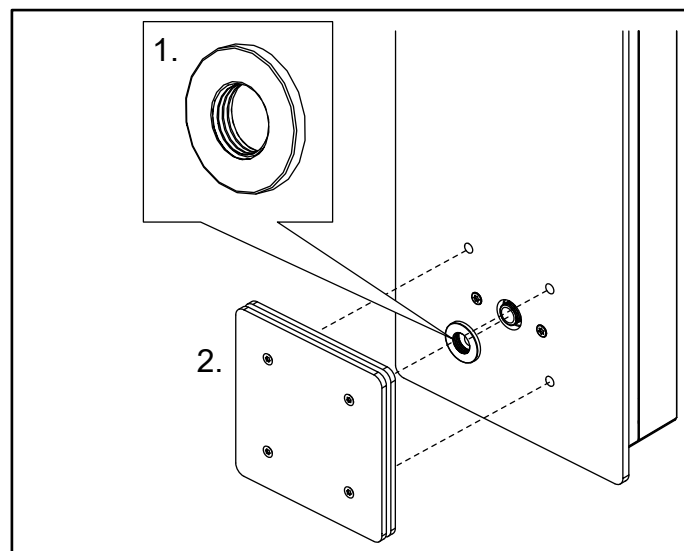
Abbildung 17 1. Die Abdeckscheibe so anschrauben, dass sie bündig zur Scheibe steht. 2. Die Dampfduüse einsetzen
