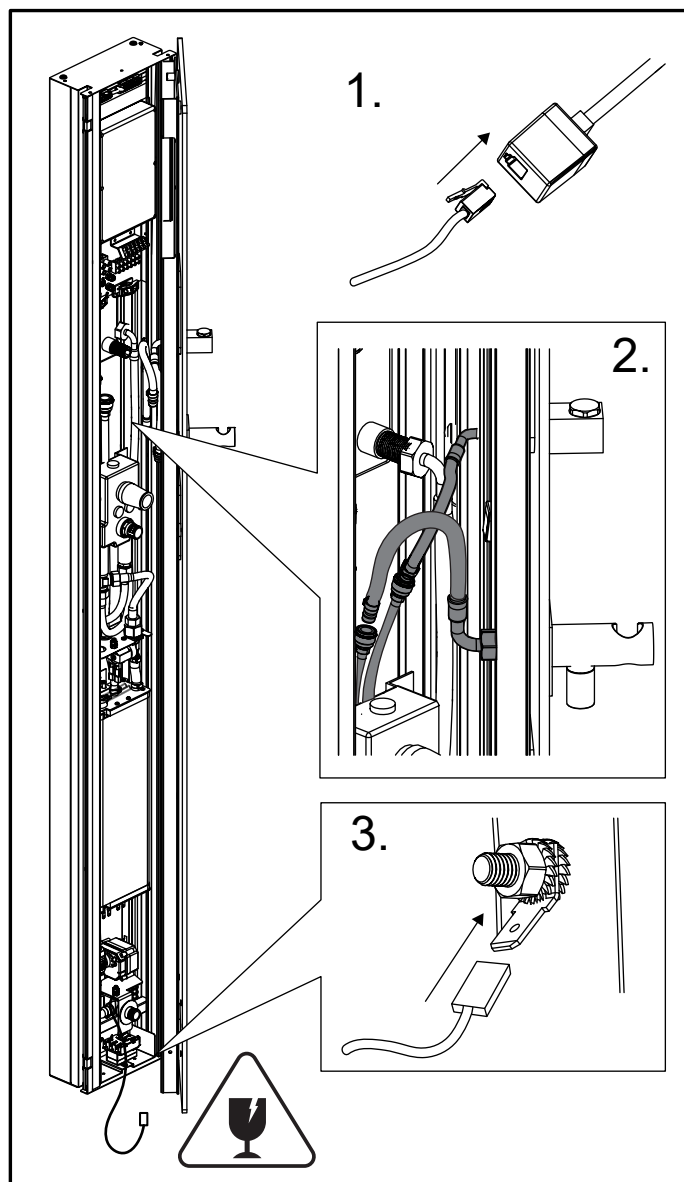
Fig. 8 Ta fronten och sätt den nära till höger om pelaren. Akta glaset. Lägg gärna en kartongbit på golvet för skydd. 1. Koppla in manöverpanelen 2. Koppla slangar, grön/gula och svarta slangen 3. Fäst jordkabel 4. Sätt på vattnet för att kontrollera att alla kopplingar är täta
