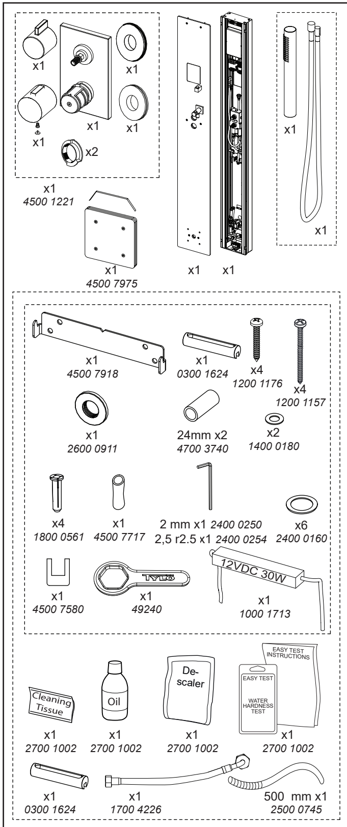
Kuva 1 Höyrypylvään osat
