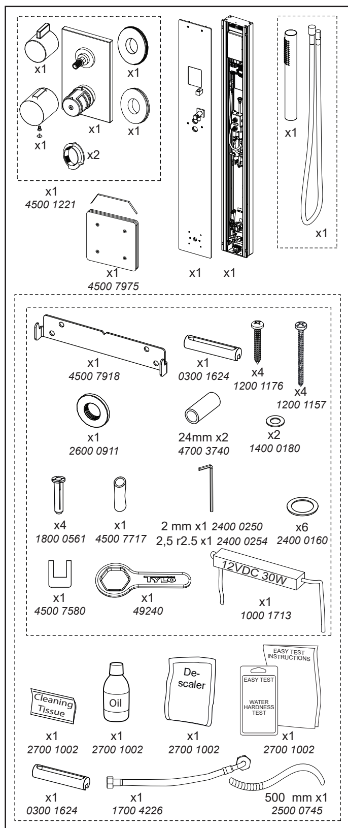
Abbildung 1: Dampfsäulenteile
