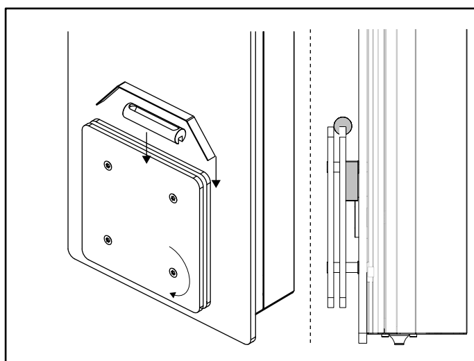
Fig. 18 Spänn de fyra skruvarna och sätt dit doftskålen och plåten för att sprida ångan längst in
