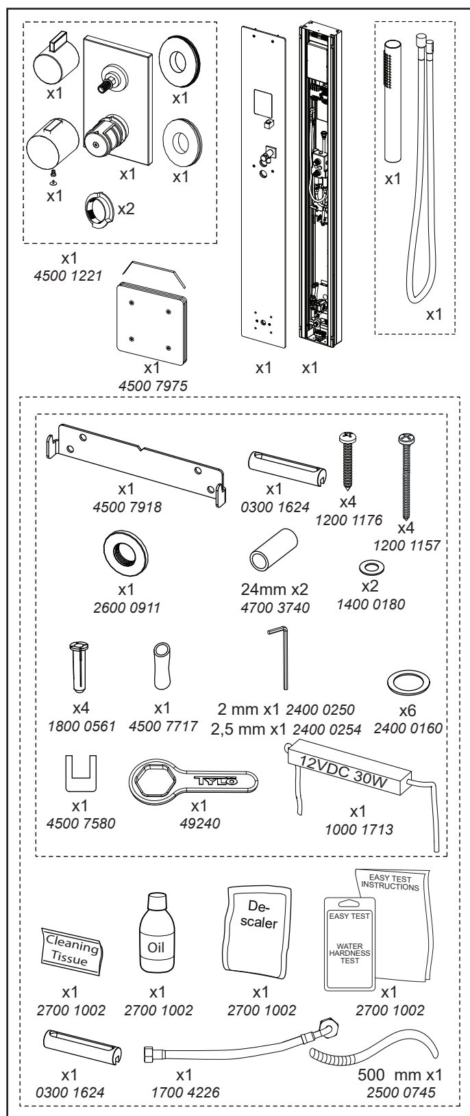
Fig. 1 Ångpelarens delar
