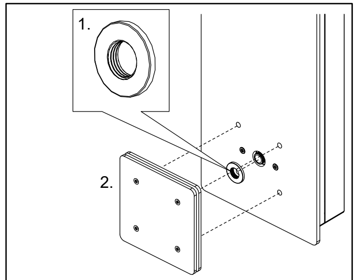
Afb. 17 1. Schroef de afdekring met de hand op zijn plaats zodat deze vlak tegen het glas aanligt. 2. Monteer het stoompijpje
