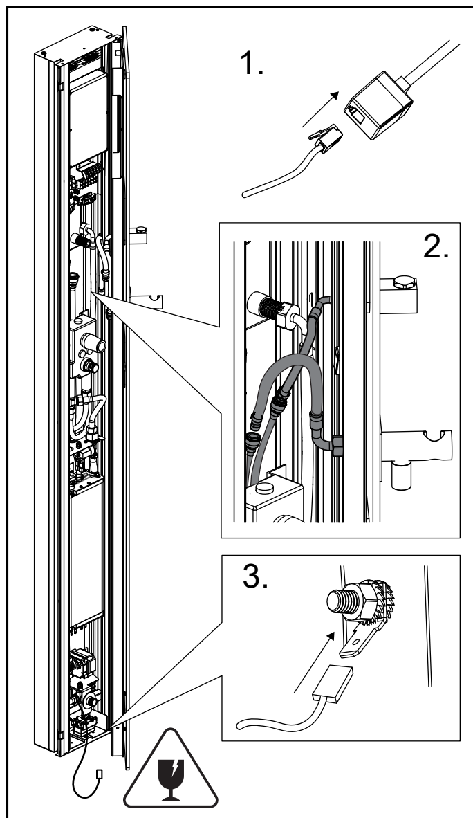
Kuva 8 Aseta etupaneeli lähelle oikeanpuoleista pylvästä. Varo lasia. Aseta tarvittaessa pahvinpala lattialle suojaksi. 1. Liitä ohjauspaneeli 2. Liitä vihreä/keltainen ja musta letku 3. Asenna maadoituskaapeli 4. Käännä vesi päälle ja tarkista, että kaikki liitännät ovat tiukat
