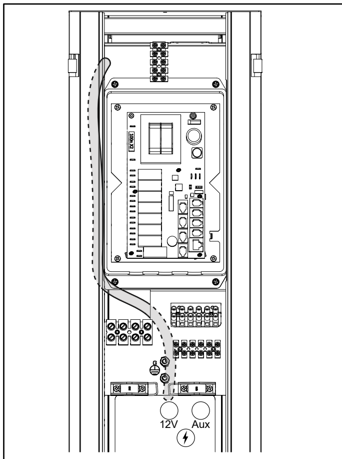
Kuva 7 Asenna joustoputki kuvan osoittamalla tavalla syöttämään LED-paneeliin 12 VDC:n virtaa
