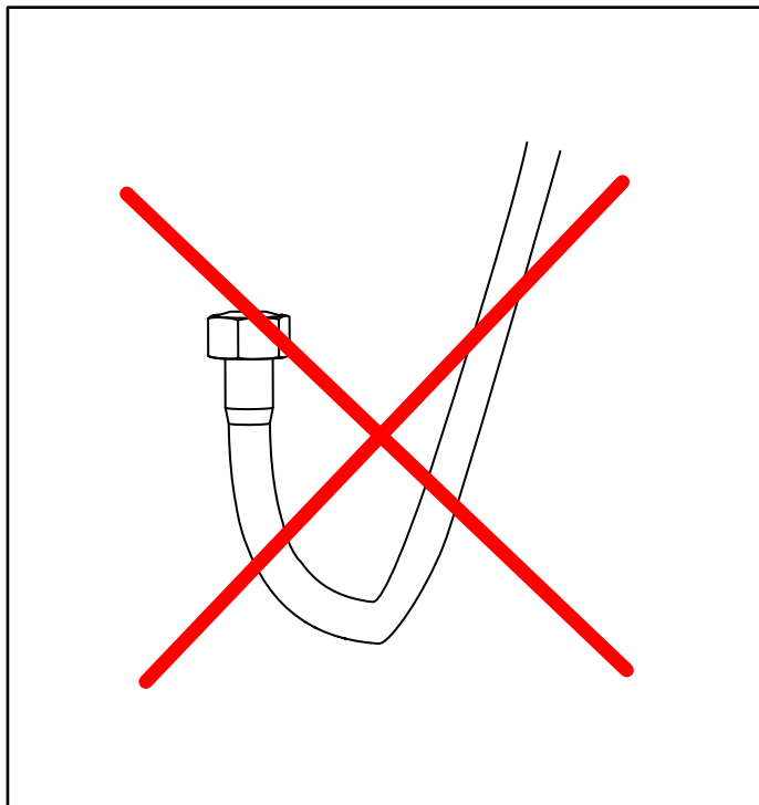
Fig. 5B Koppla in varmt och kallt vatten. Vrid slangarna så att inga knäckar bildas. Skruva åt. Sätt på vattentryck för att kontrollera tätheten.
