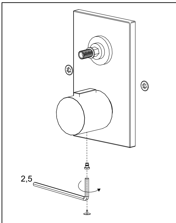
Fig. 15 Lås termostadvredet och tryck på täcklocket
